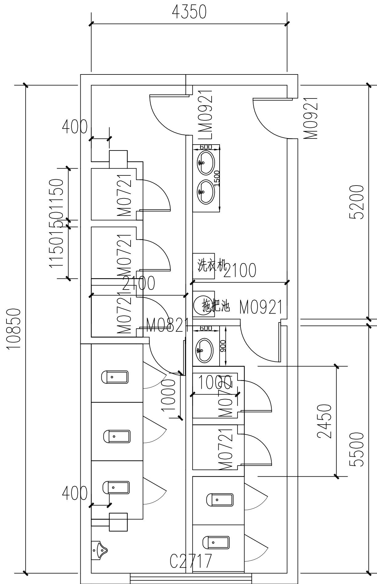
二楼卫生间改造
